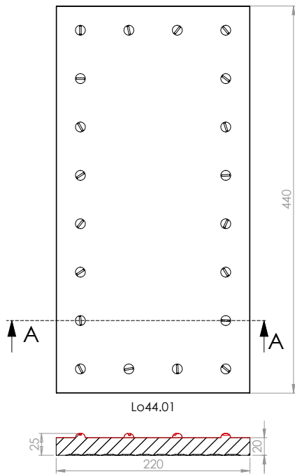
PRZEKRÓJ A-A
