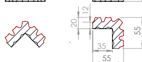
PRZEKÓJ A-A
