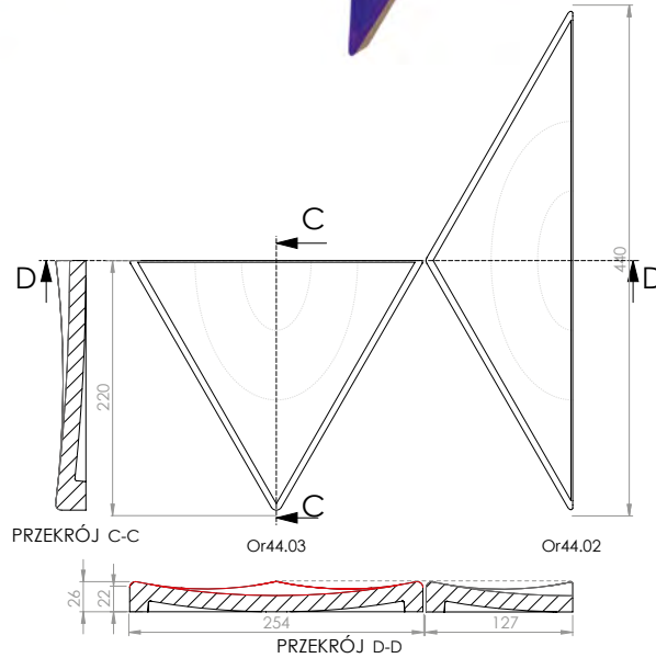
PRZEKRÓJ D-D
