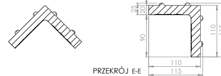
PRZEKÓJ E-E
