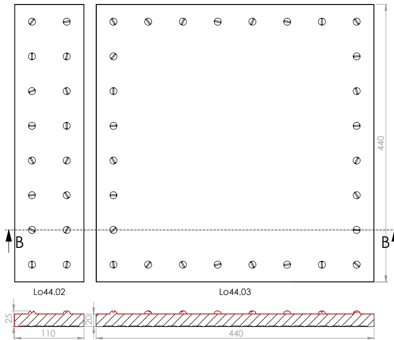
PRZEKRÓJ B-B
